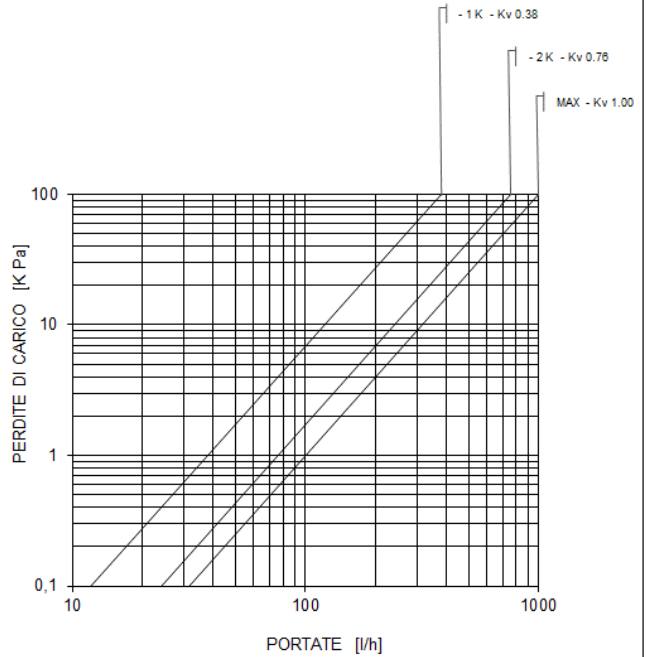
Corpo a squadra con attuatore ATW 130UM - VSQ34FW-PR DN 3/4" Preregolazione SP 3
