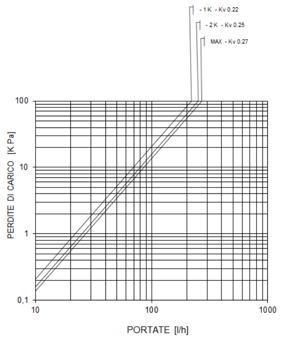
Corpo a squadra con attuatore ATW 130UM - VSQ34FW-PR DN 3/4" Preregolazione SP 1
