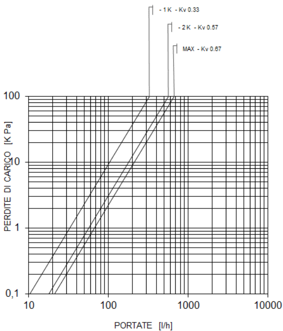
Corpo a squadra con attuatore ATW 130UM - VSQ34FW-PR DN 3/4" Preregolazione SP 2
